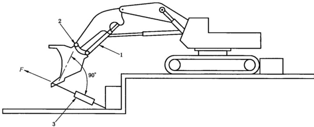
b) 正铲液压挖掘机
