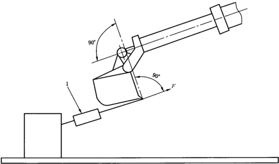
标号： F ——挖掘力； 1——测力计(载荷传感器)。
